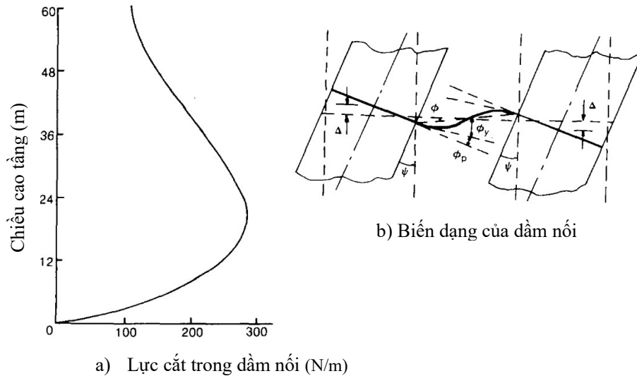
Hình 2. Lực cắt phân bố và biến dạng trong dầm nổi (J.S Kuang [5])
