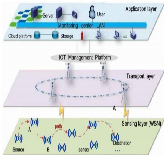
شکل (۱): سناریوی ساده شده یک شبکه حسگر بی سیم در [2] IOT
