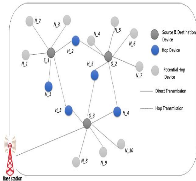
شکل (۲): معماری مدل انتخاب هاپ کارآمد انرژی برای شبکه حسگر [3]
