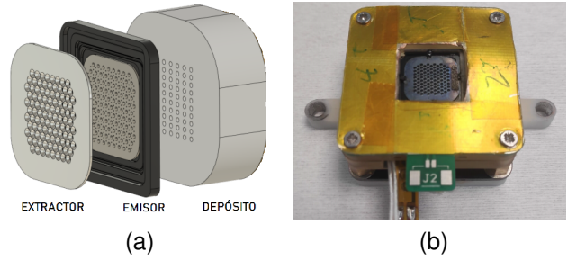
Figura 3. Cabecal del propulsor ATHENA-XM0. (a) Vista explosionada. (b) Montaje experimental.
